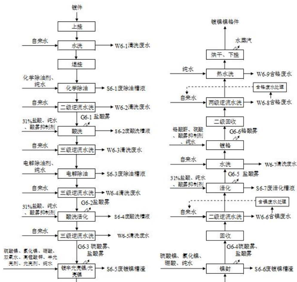
图4.1-4 镀镍镍铬生产工艺流程图
