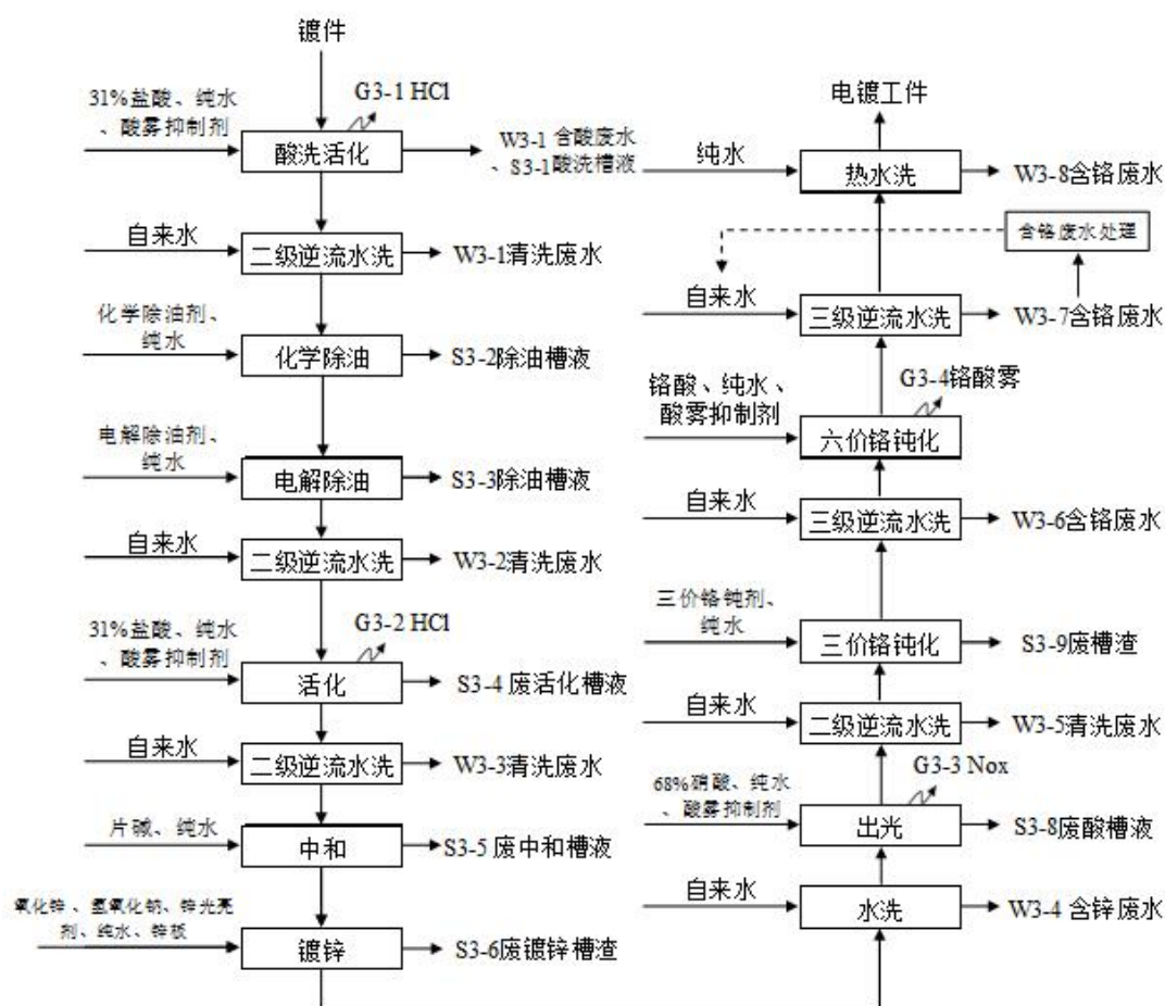
图 4.1-2 碱性镀锌生产工艺流程图
