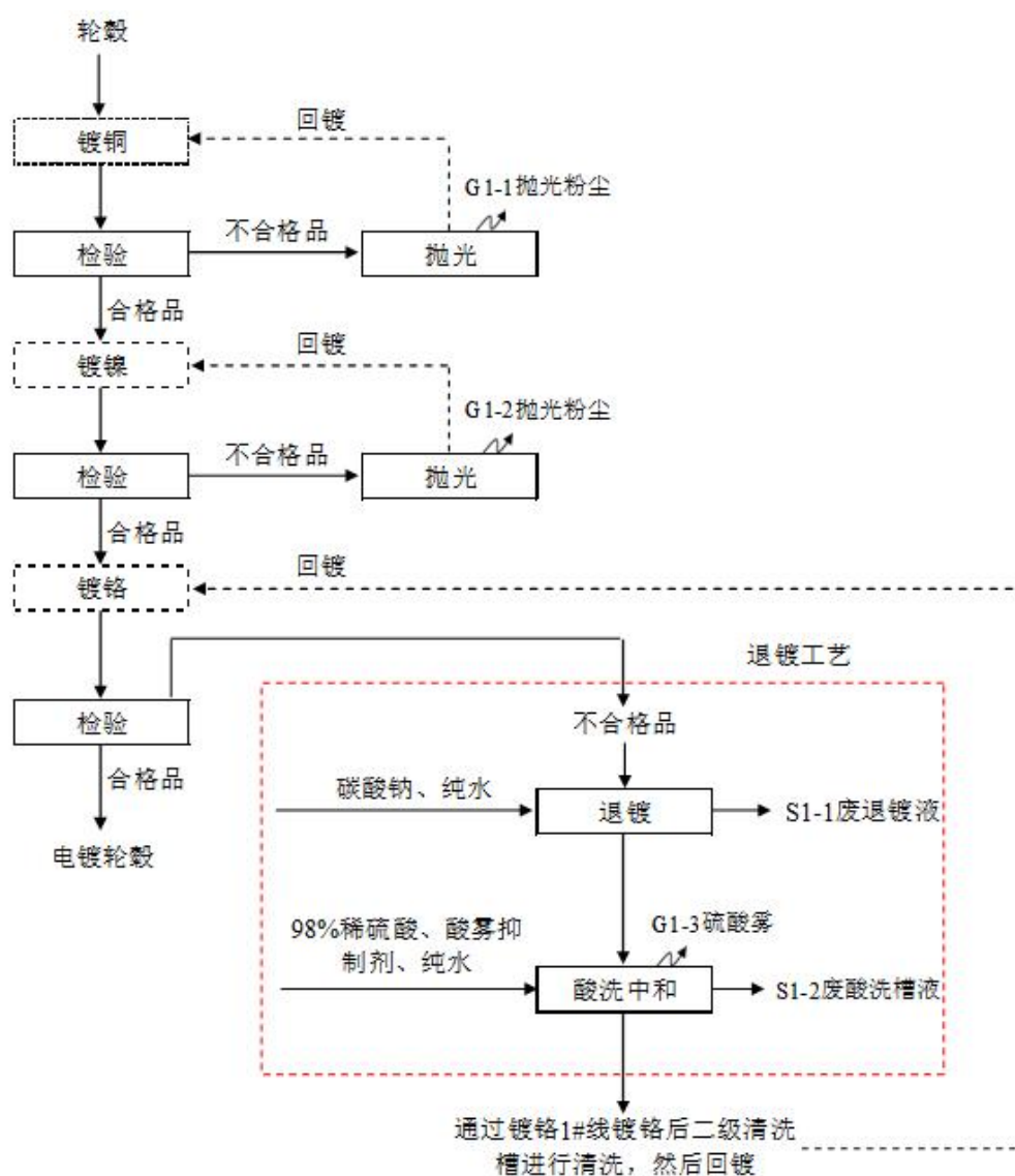
图4.1-1 镀铜镍铬总体工艺流程图
