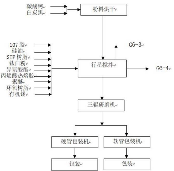
图 4.1-7 高性能密封材料生产工艺流程图
