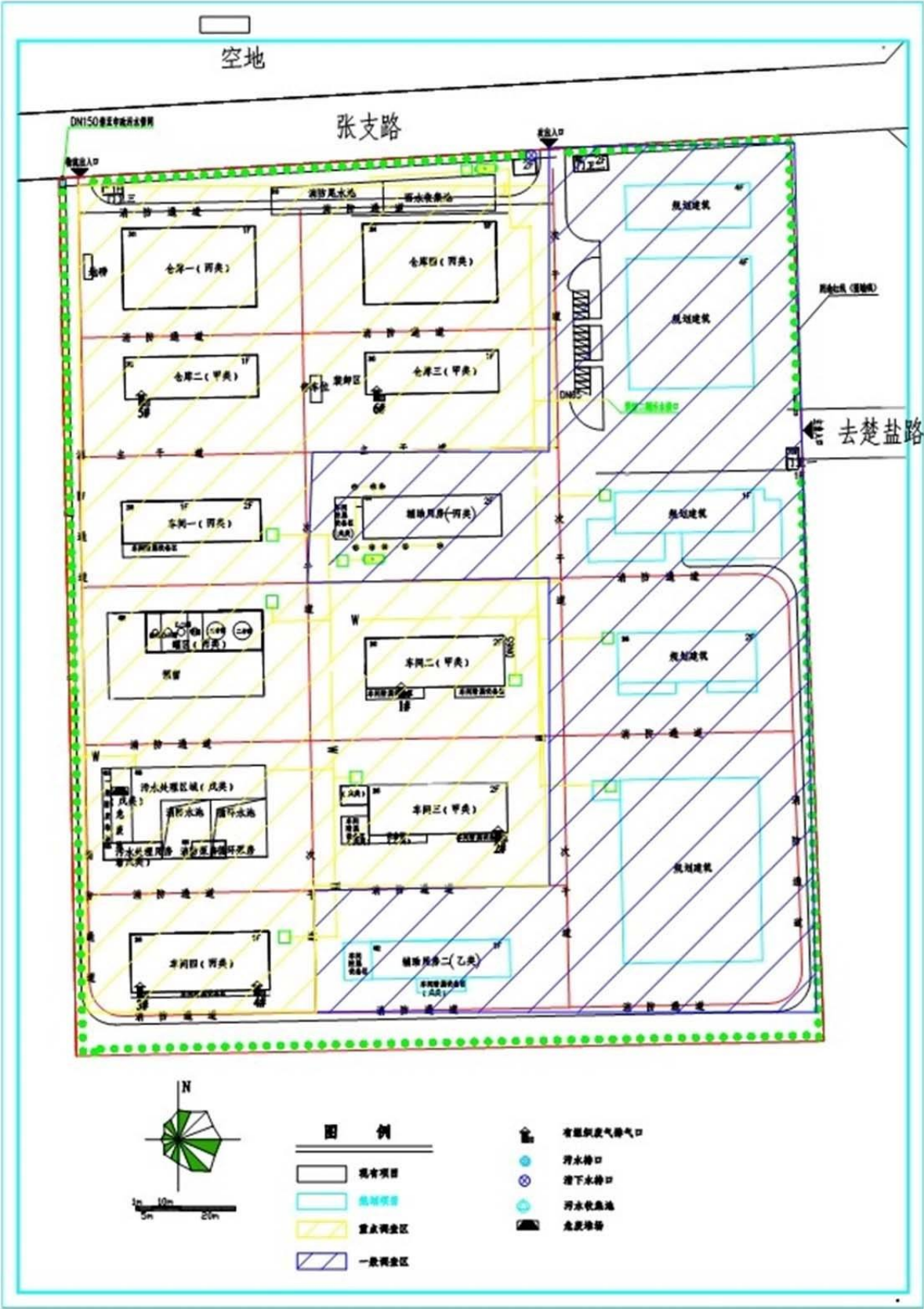
图 5.2-1 瑞洋安泰厂区分区图
