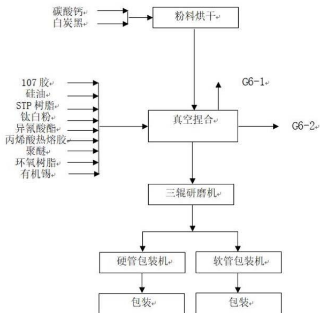
图 4.1-6 高性能密封材料生产工艺流程图
