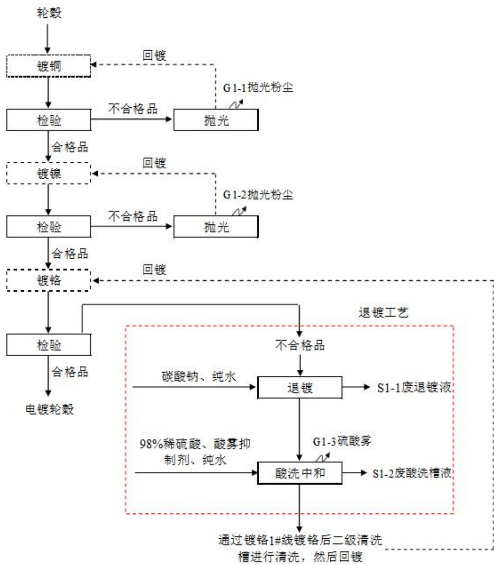
图4.1-1 镀铜镍铬总体工艺流程图
